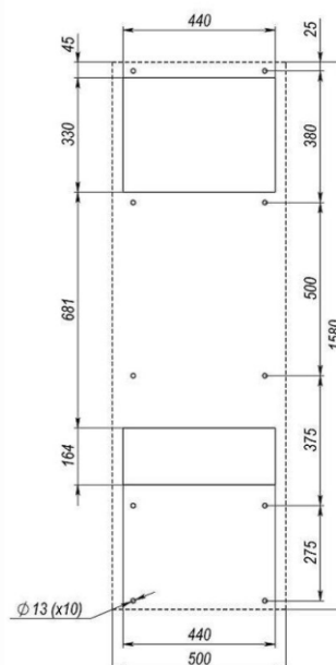
Наружный монтаж
