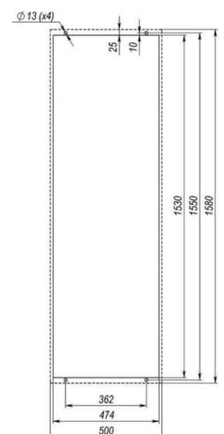
Полутопленный монтаж
