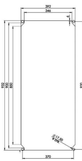
Монтажный вырез полуутопленный монтаж
