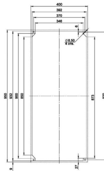
Монтажный вырез утопленный монтаж
