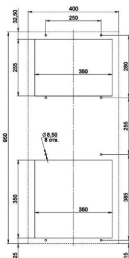
Монтажный вырез наружный монтаж
