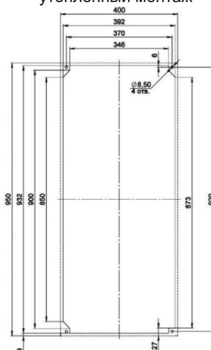
Монтажный вырез утопленный монтаж
