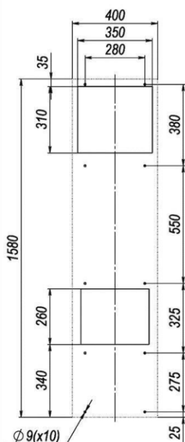
Монтажный вырез наружный монтаж
