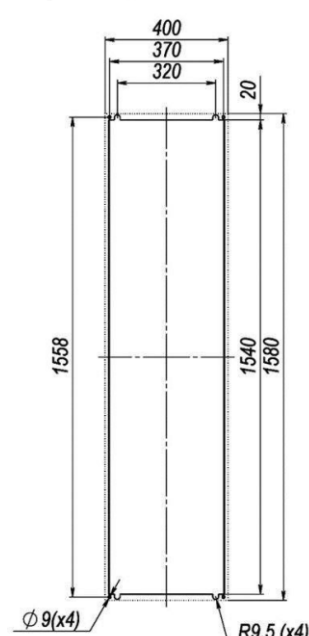
Монтажный вырез полуутопленный, утопленный монтаж
