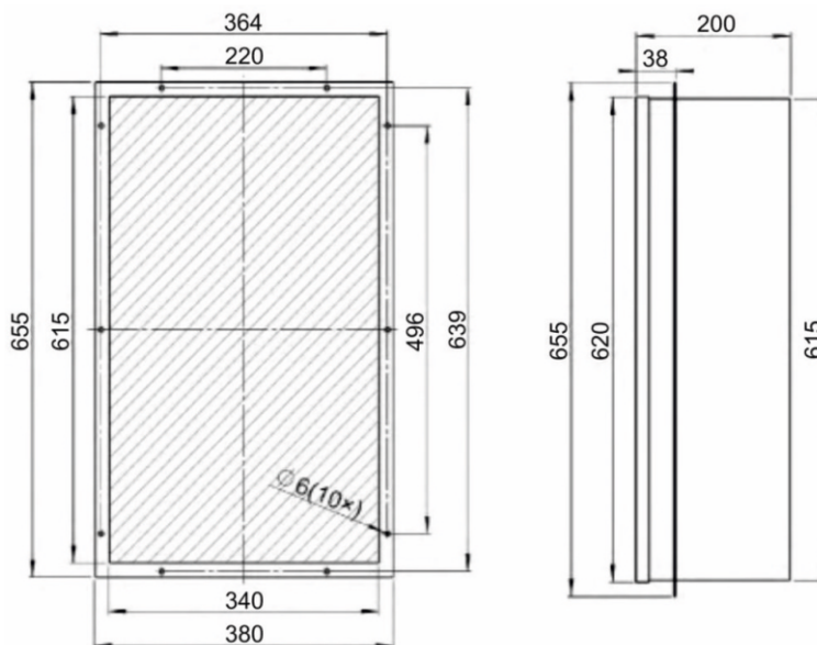
ЧЕРТЕЖИ ПРИСОЕДИНИТЕЛЬНЫХ РАЗМЕРОВ UNISPLIT NS-500(1)W
