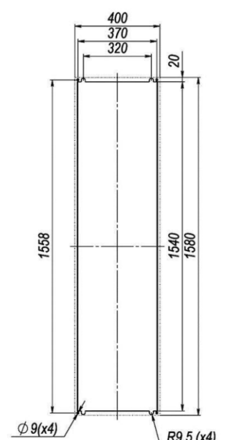
Монтажный вырез полуутопленный, утопленный монтаж
