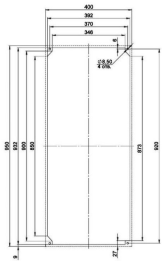
Монтажный вырез утопленный монтаж
