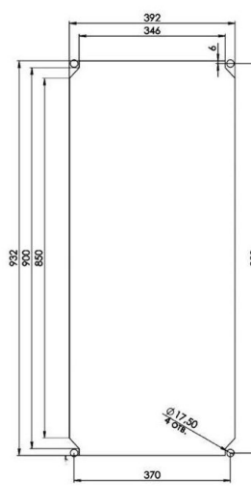
Монтажный вырез полуутопленный монтаж
